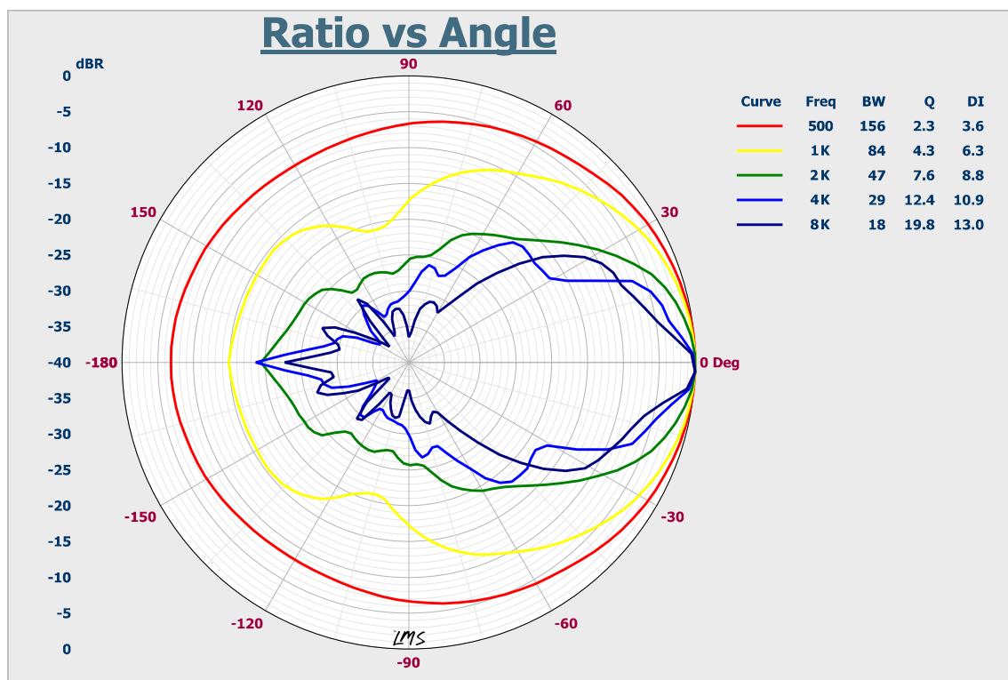
Круговая диаграмма направленности громкоговорителя LPA-50H
